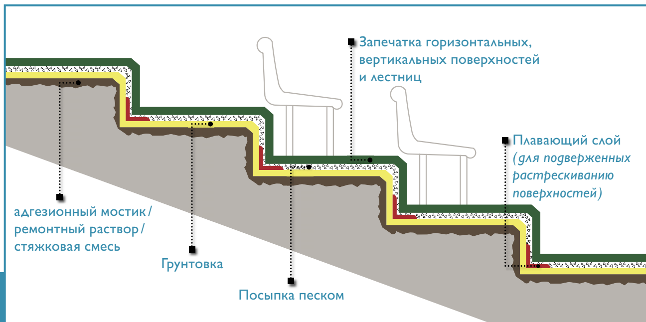
Схема системы - "Санирование трибун для зрителей"
