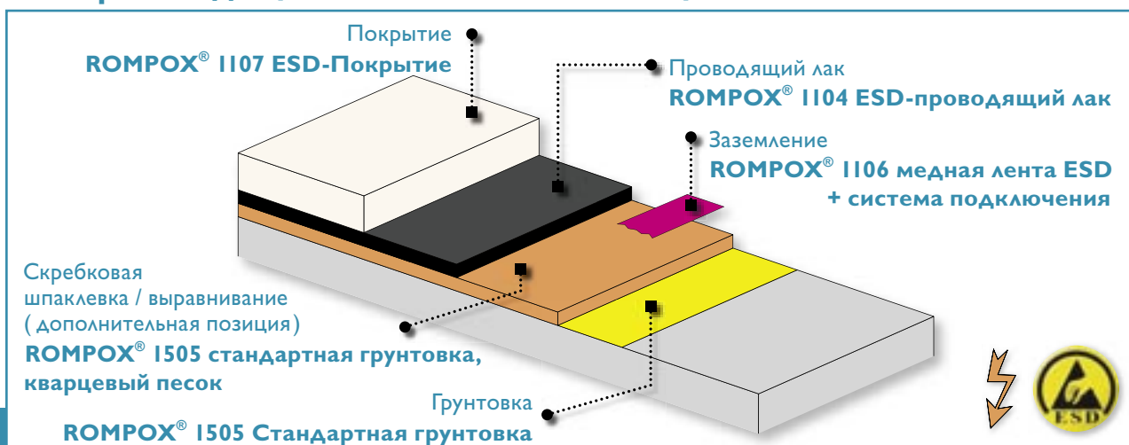
Система "Покрытие для чистого помещения с покрытием ROMPOX® 1107 ESD" (отводящее электростатику)
