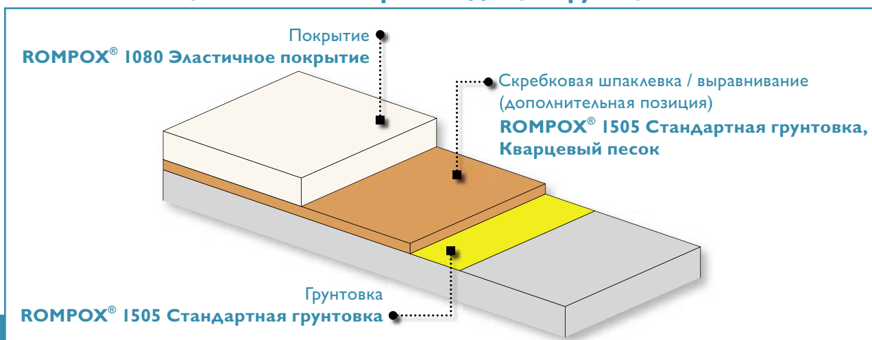
Система “Покрытие для чистого помещения с эластичным покрытием ROMPOX® 1080 “ (без электроотводности)
