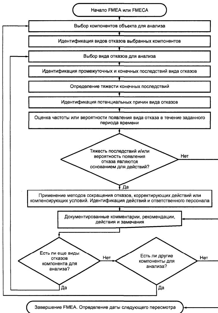
Рисунок 2 - Блок-схема анализа
