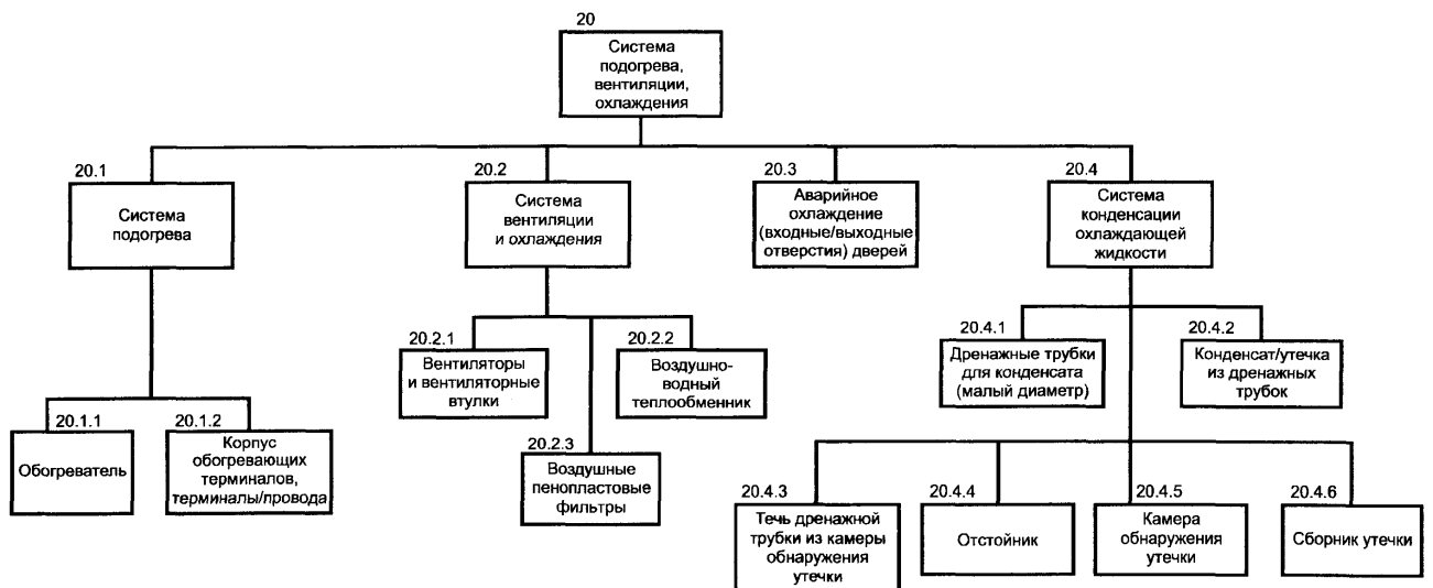
Рисунок В.3 - Диаграмма системы нагревания, вентиляции, охлаждения
